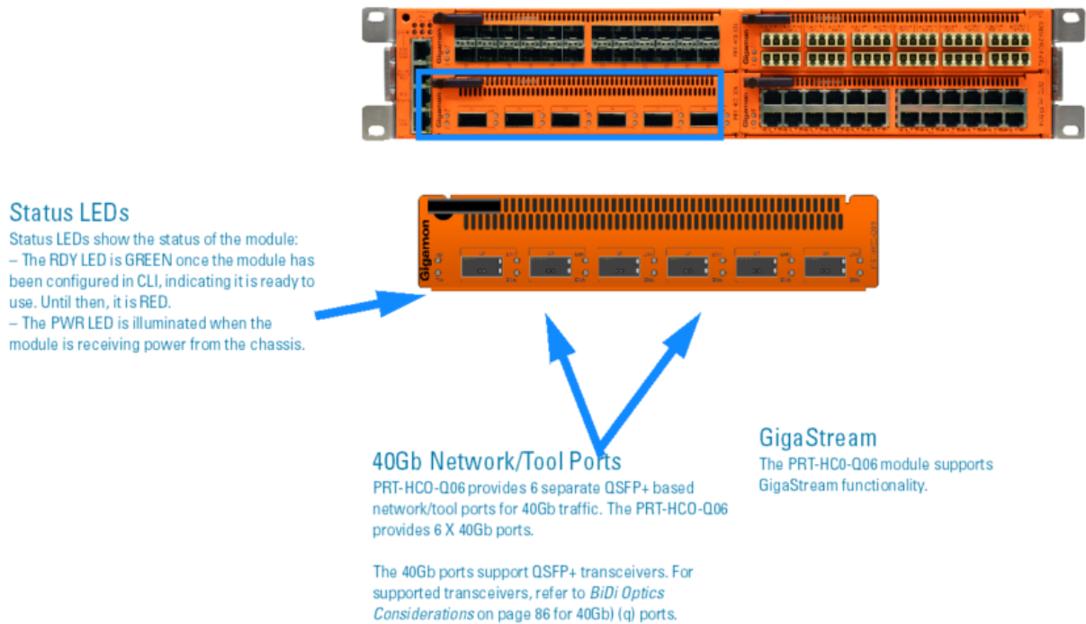
Figure 5 PRT-HC0-Q06 Module
